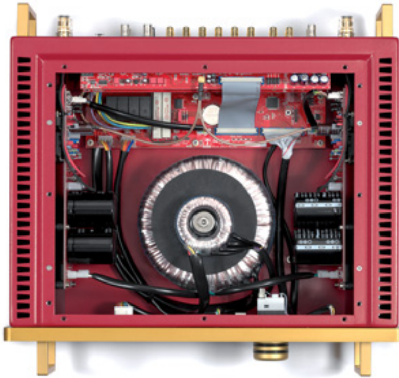
Vier Hanteln, drei Füße, zwei Trafos: Auch aus mechanischer Sicht ist der Dartzeel ein Traum. Patentiert: die Minimalschaltung. Nicht patentiert: die Farbgebung
