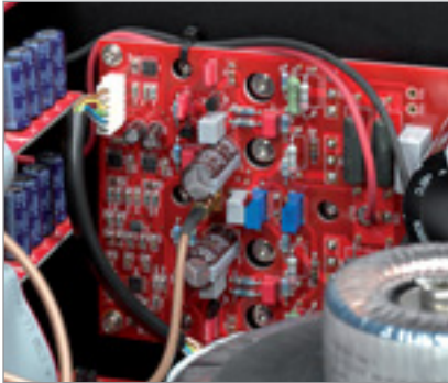
Vier Leistungstransistoren pro Kanal: diskret aufgebaute Endstufenblöcke
